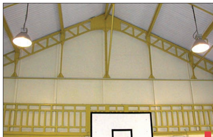
La charpente métallique du gymnase Gustave Bienvêtu.
